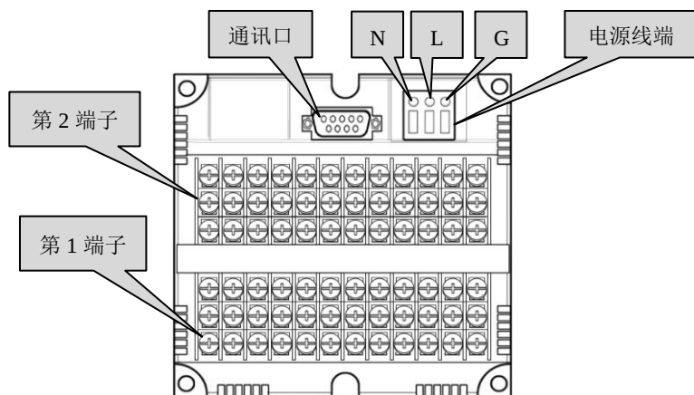
图 2-2-3-A 端子排列图
