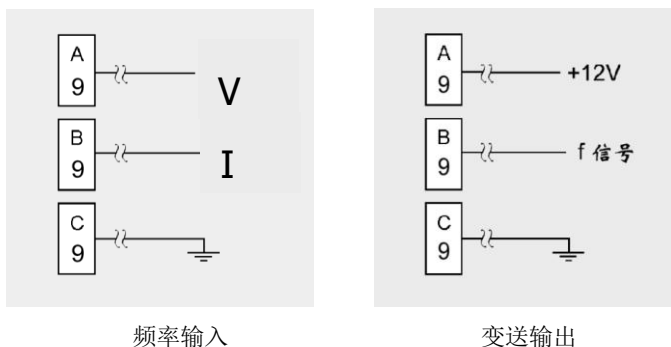
图 2-2-5 频率输入、变送输出接线图
