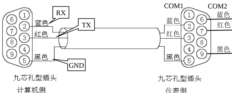
图 2-2-7-A 计算机与仪表间的 RS-232C 通讯线
